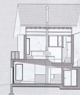
Dachgeschoss Südöstlich
