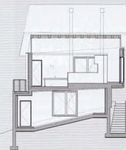
Querschnitt Nordwestlich
